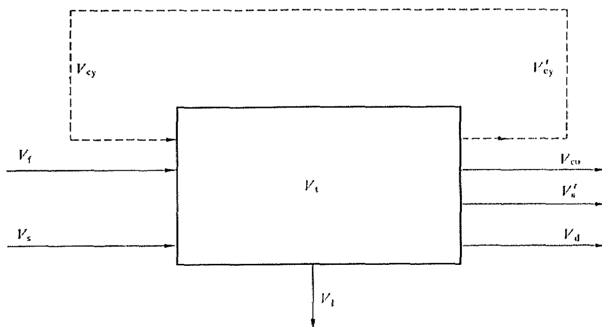
图 2 水平衡基本图示
